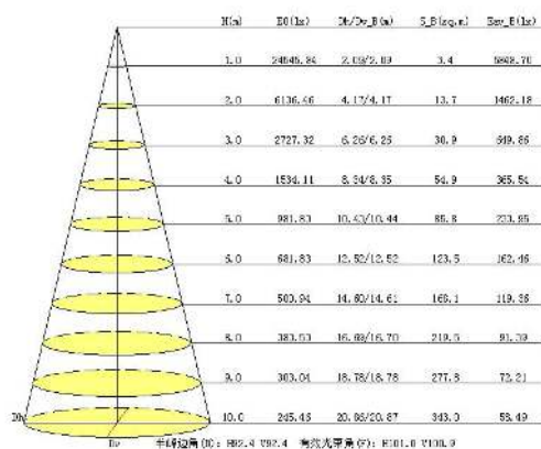
照度距离关系图
