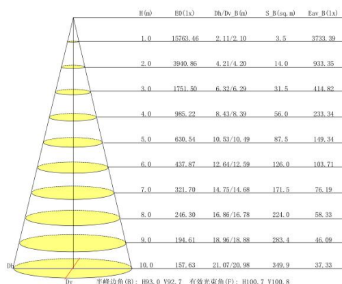
照度距离关系图
