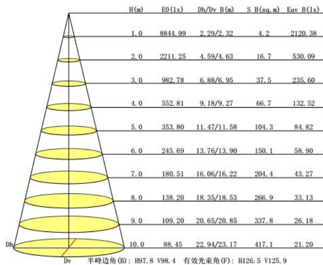
距离照度曲线
