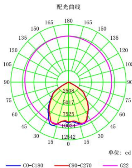
200W 流通型工矿灯-110° 灯罩
